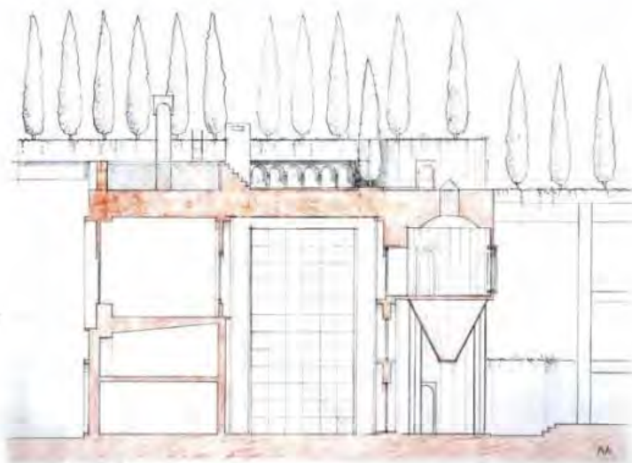
Один из чертежей с планом озеленения фабрики
